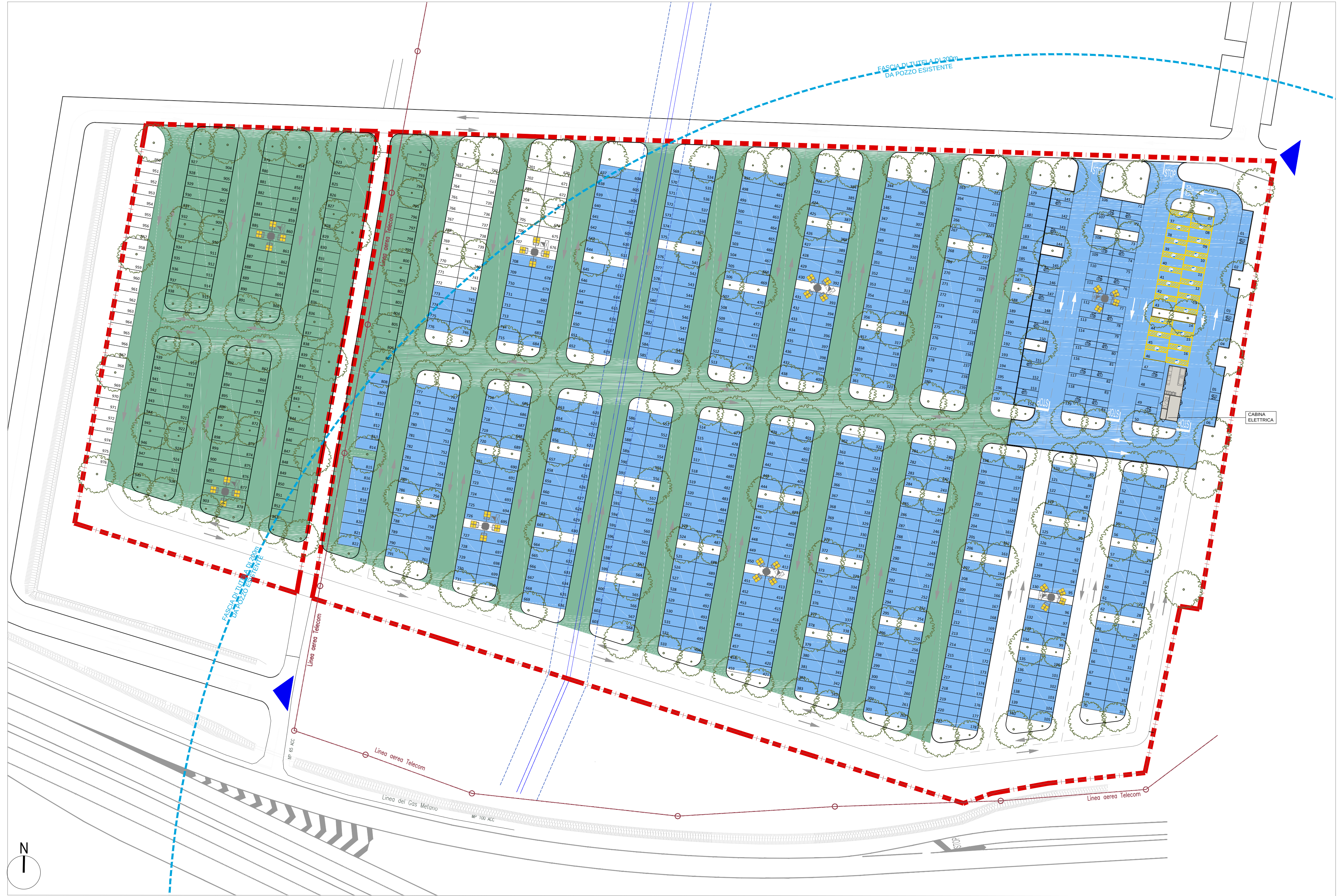
Planimetria generali dei materiali 1:500
