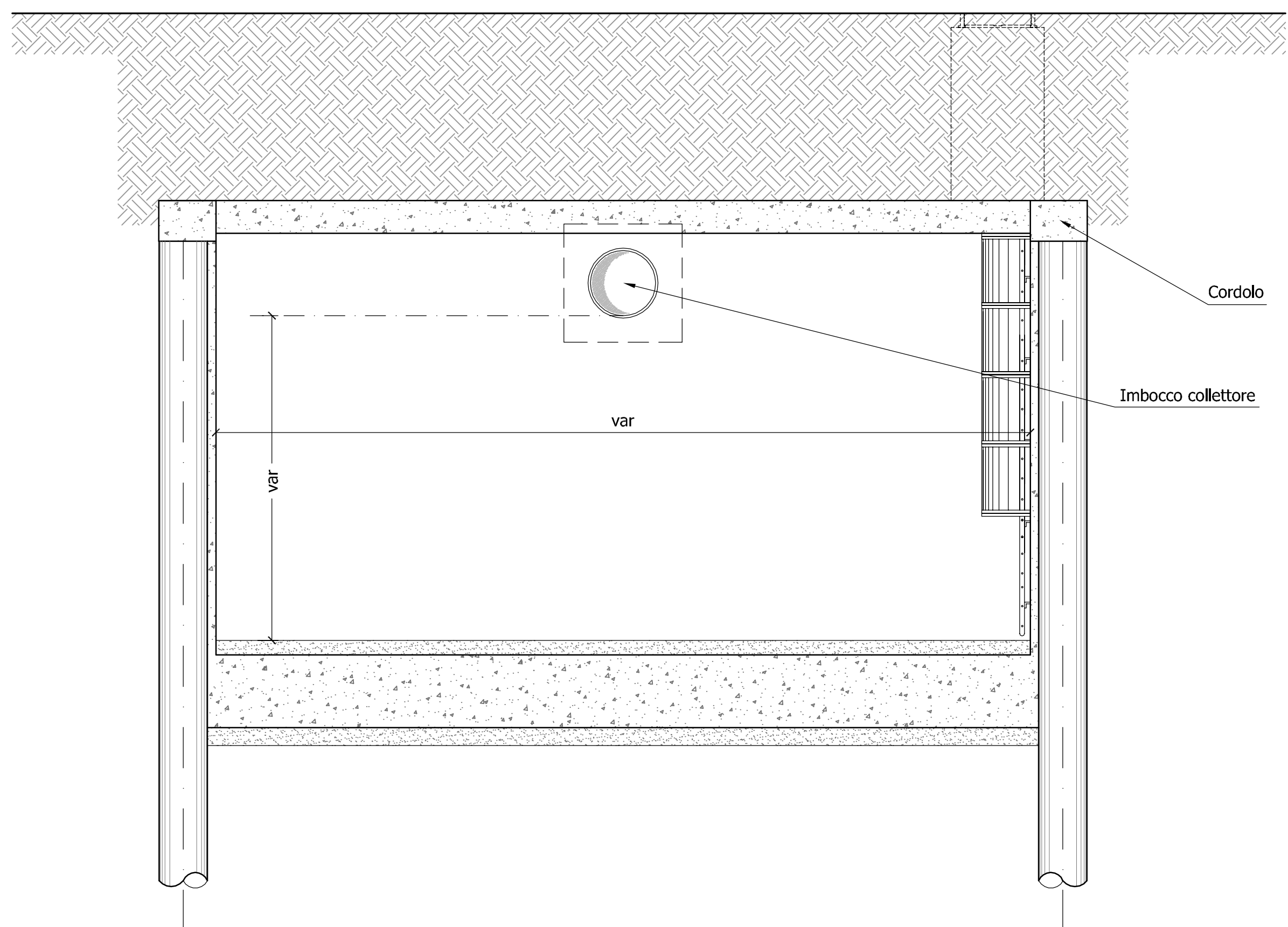
Sezione CC
