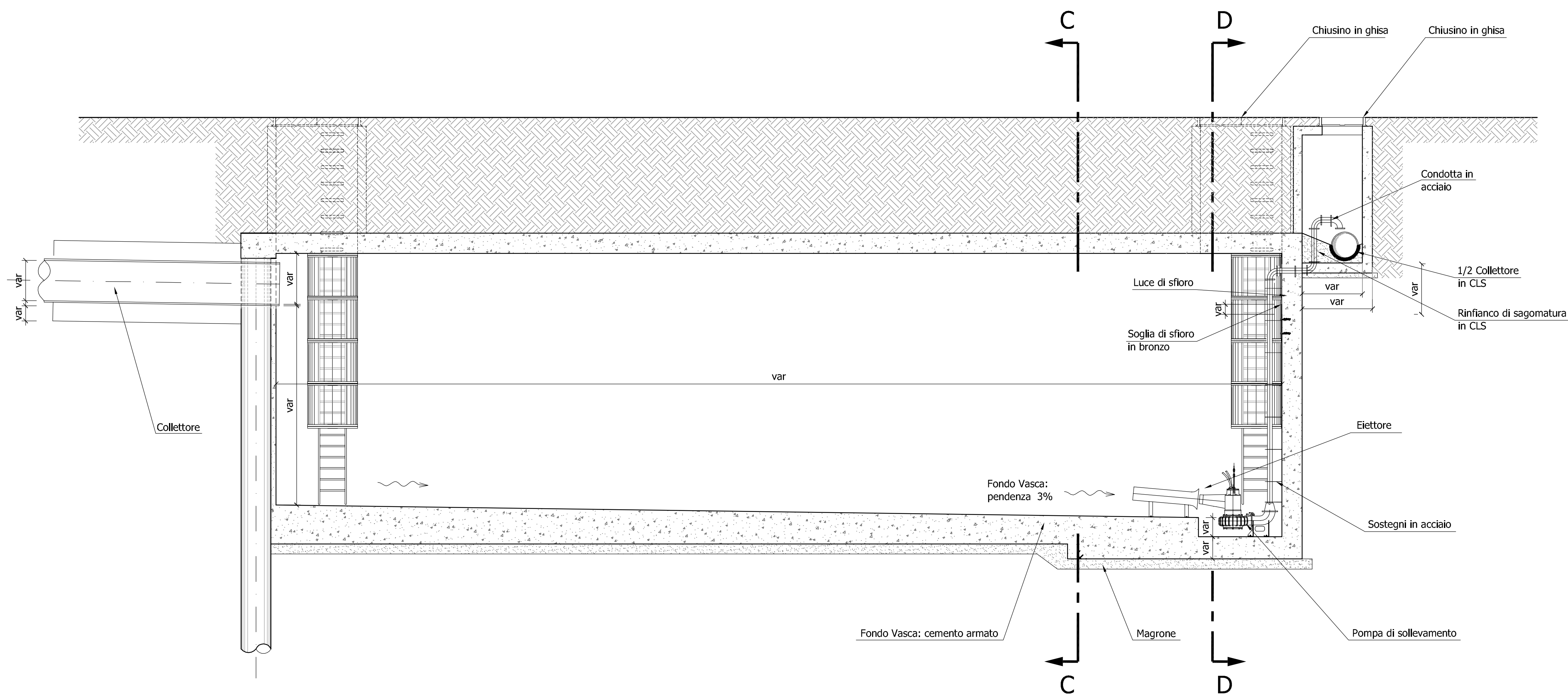
Sezione AA
