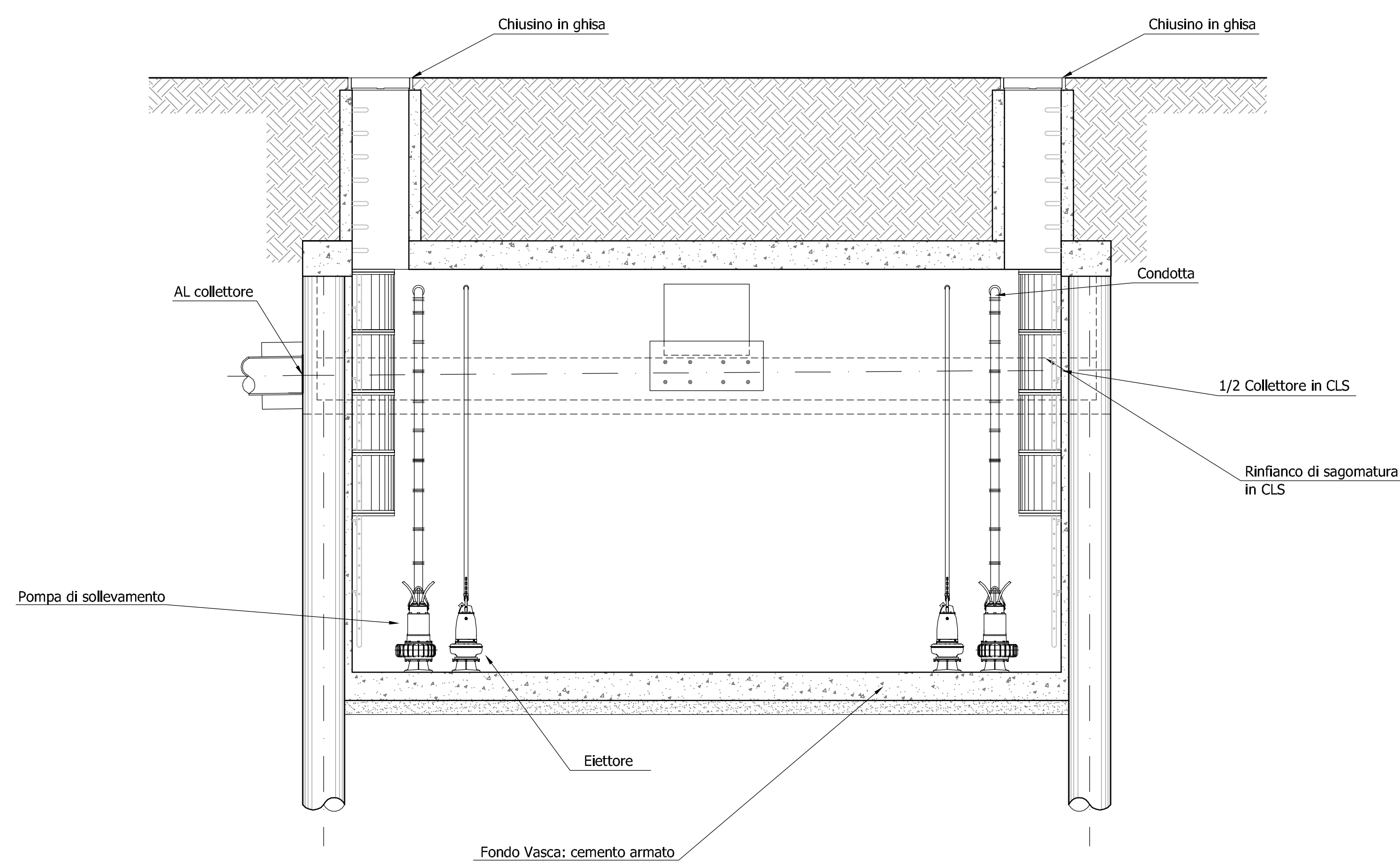
Sezione DD
