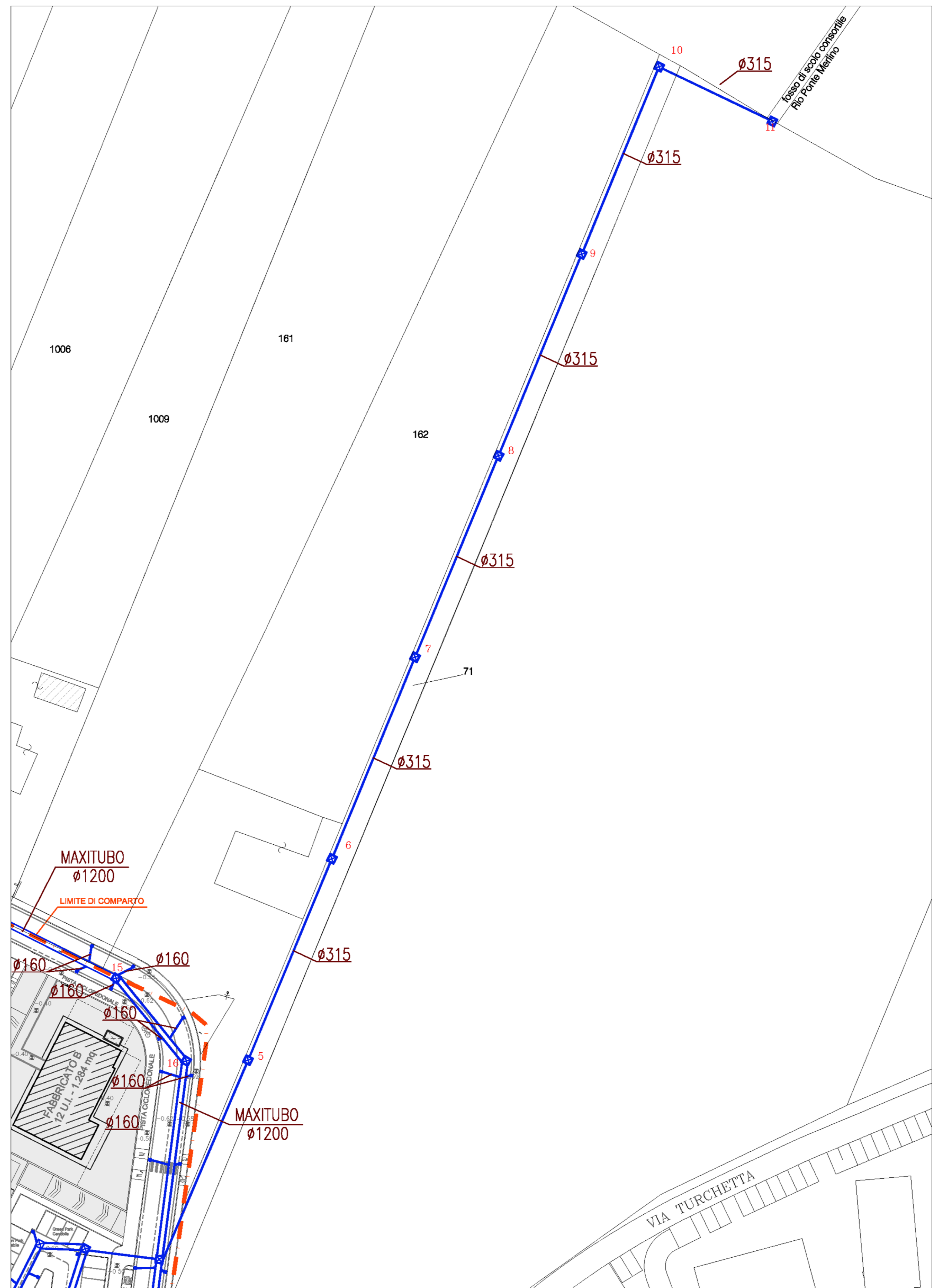
PLANIMETRIA GENERALE - QUADRO 2 - SCALA 1:500
