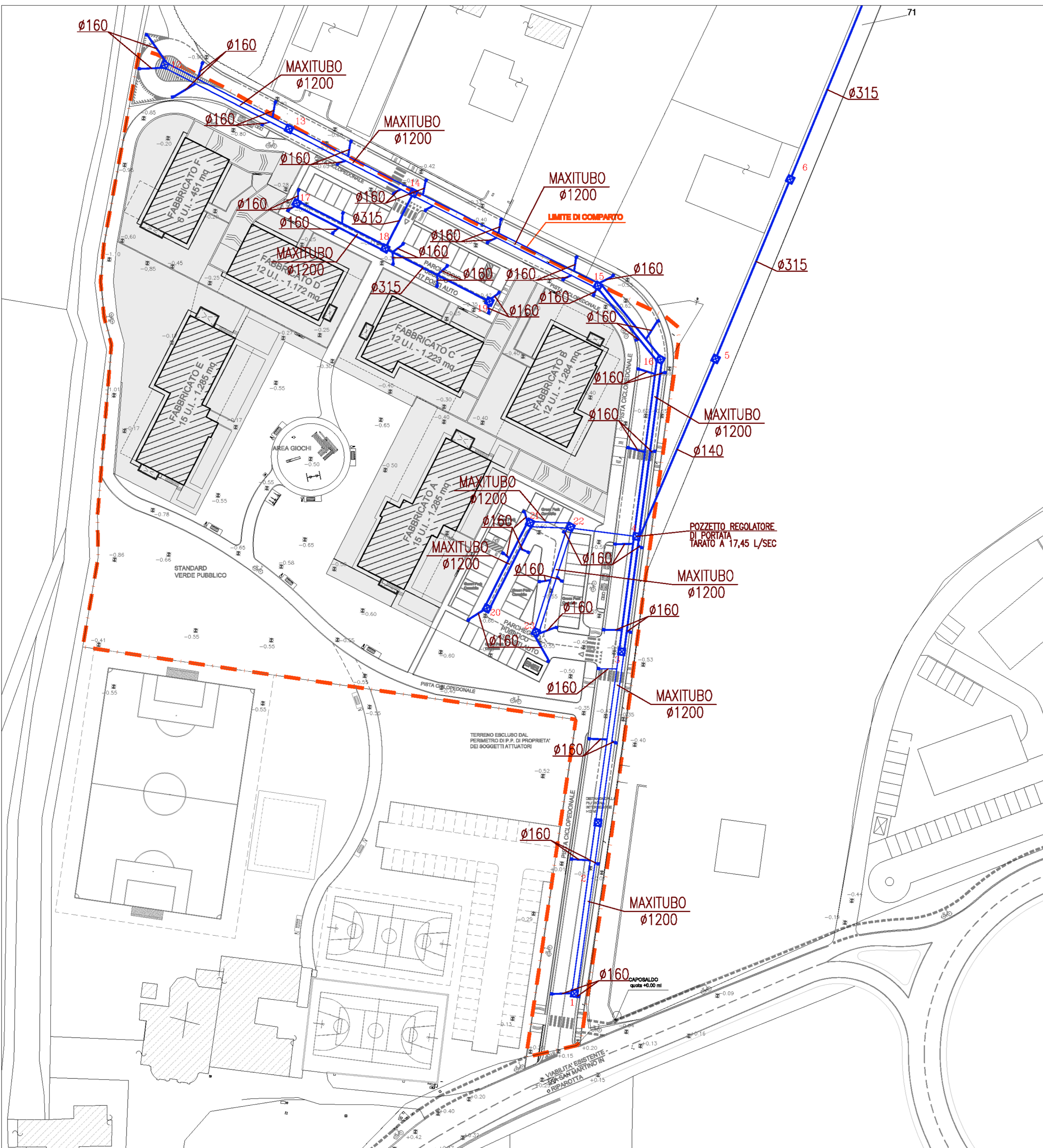
PLANIMETRIA GENERALE - QUADRO 1 - SCALA 1:500
