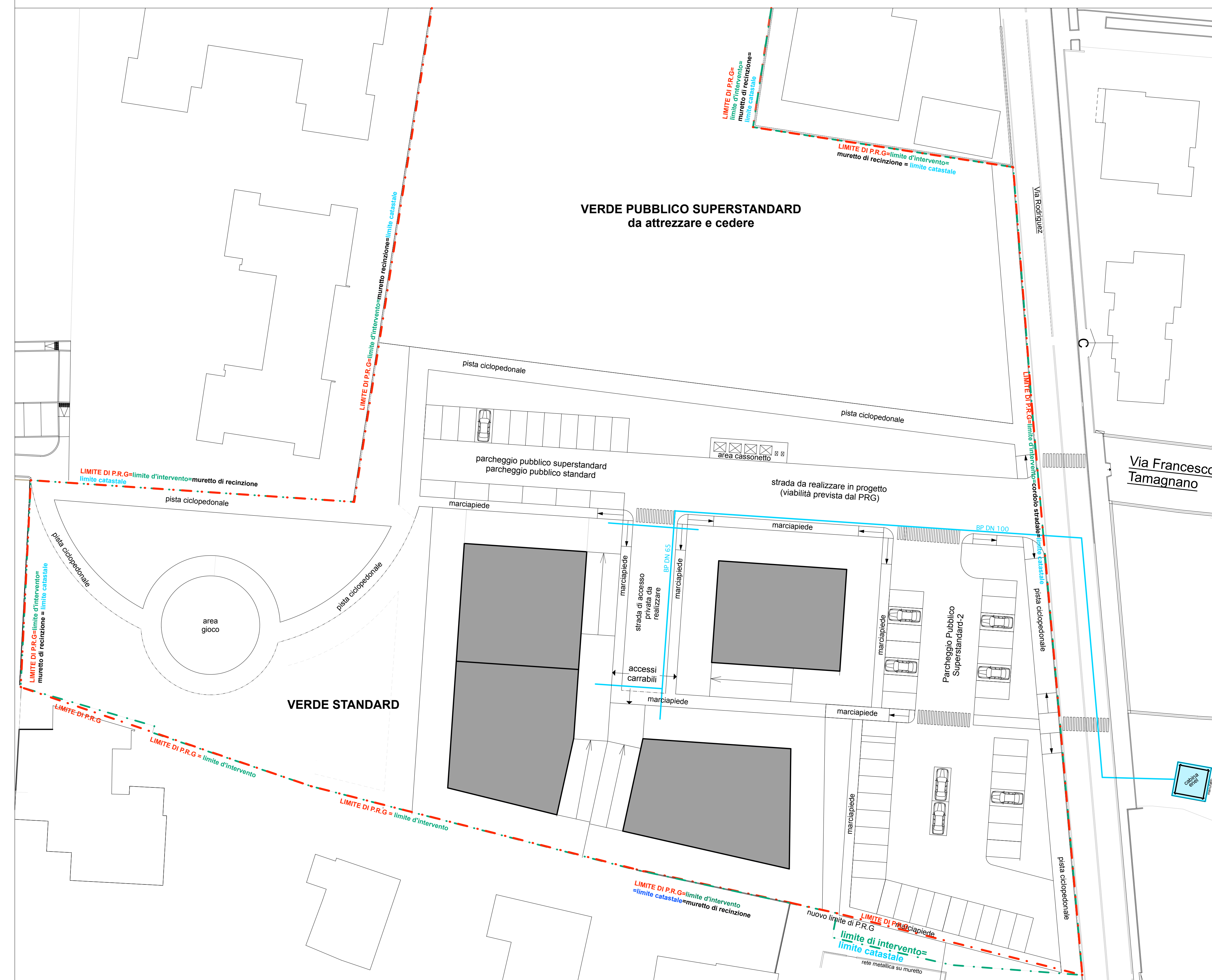
PARTICOLARE RETE ENEL scala 1:20
