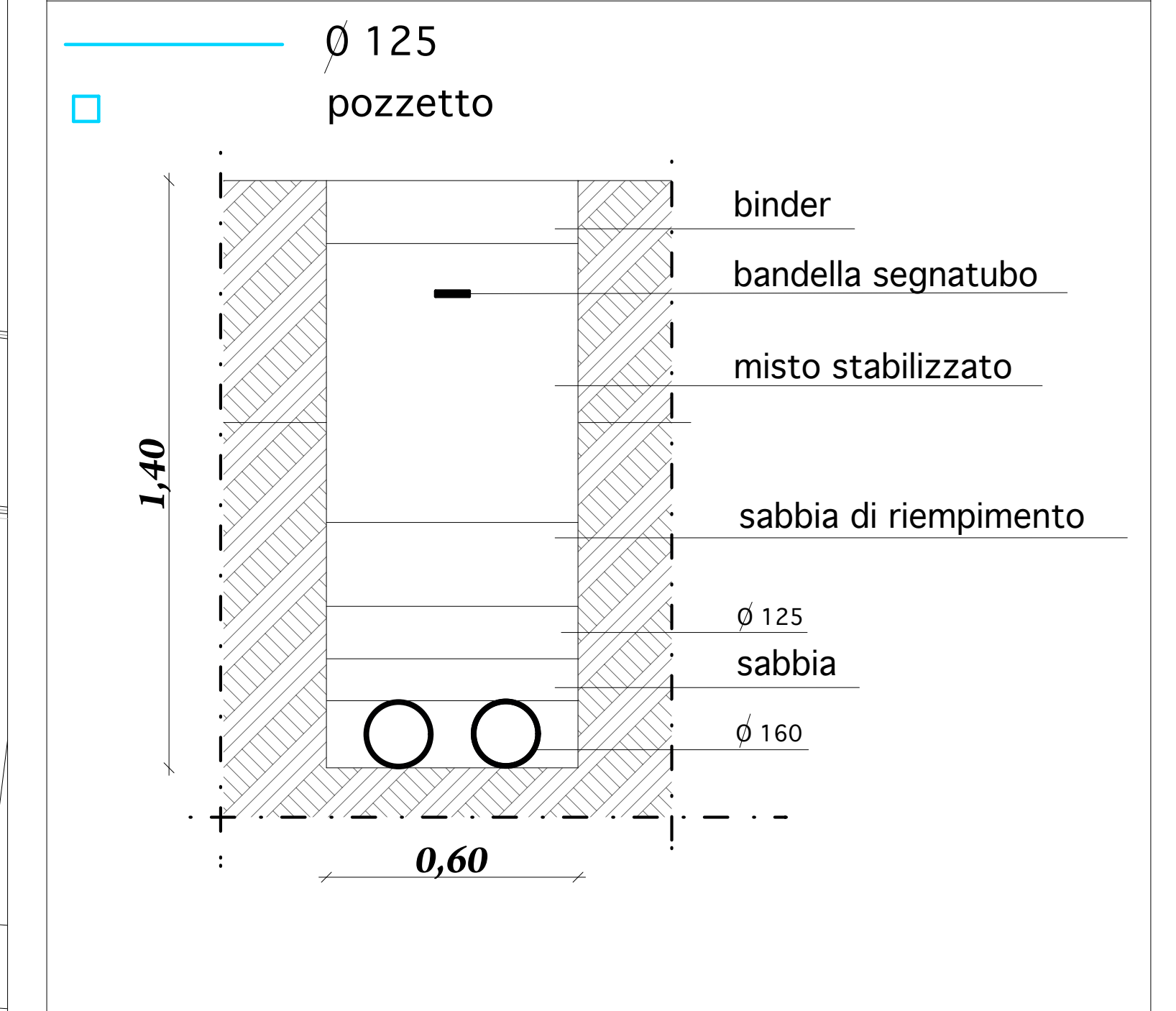
PARTICOLARE RETE ENEL scala 1:20
