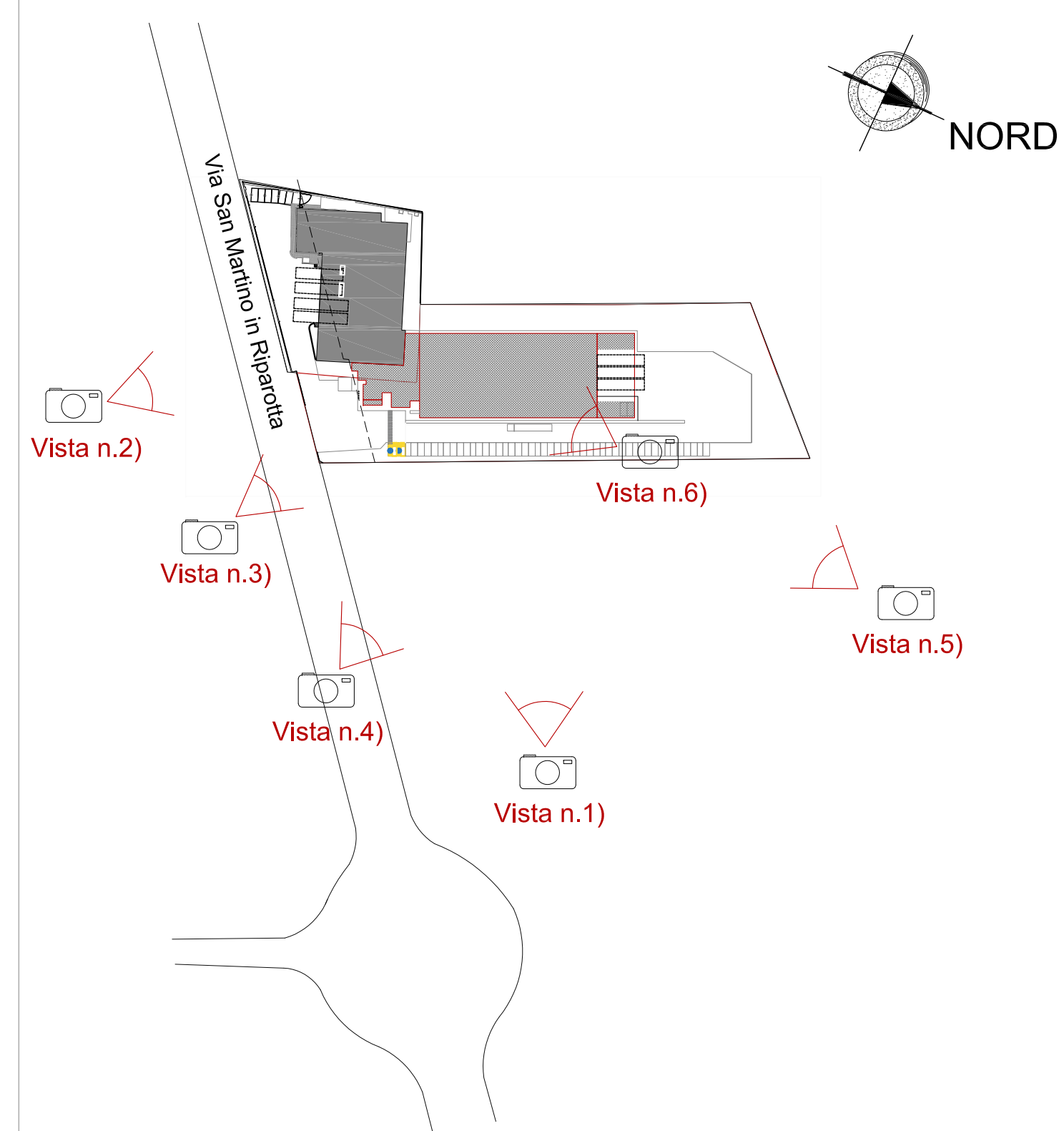
Planimetria di Progetto con punti di vista tridimensionali
